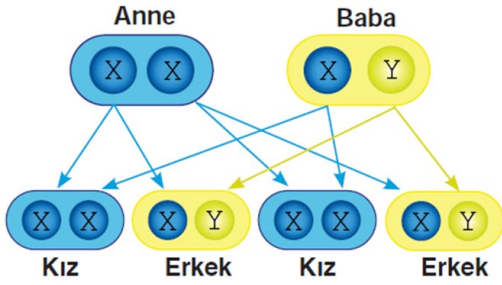
Dişi bireyin kromozom gruplandırılması: 44 + XX
